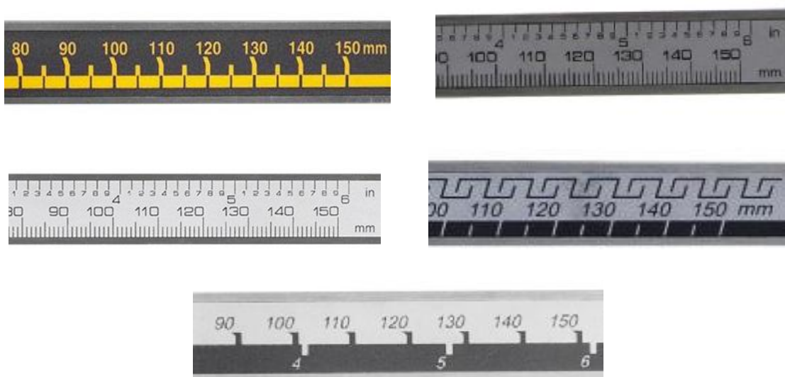
Рисунок 9 – Внешний вид штанги штангенциркулей ШЦЦ с оцифровкой
